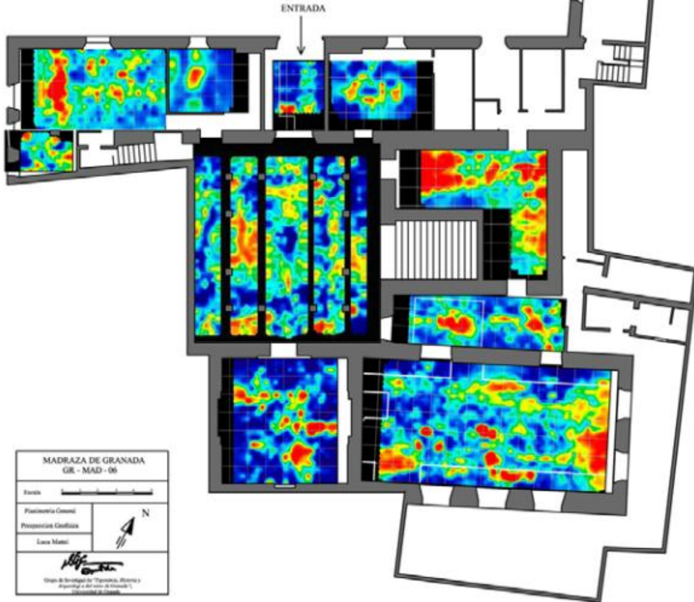
Lám. 1. Resultados de la prospección geofísica
